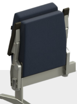
Piede anti-ribaltamento con registri Anti-tilt foot with registers
