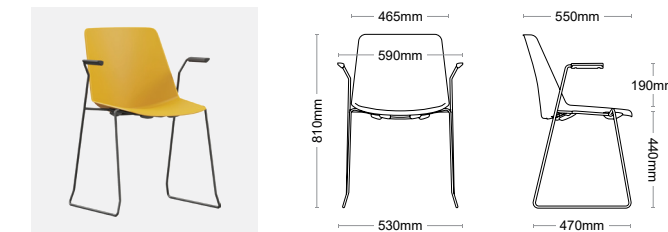
F Piramidal c/ Apoio de Braço - Pyramidal with Armrest Piramidal con reposabrazos - Pyramidal avec accoudoir
