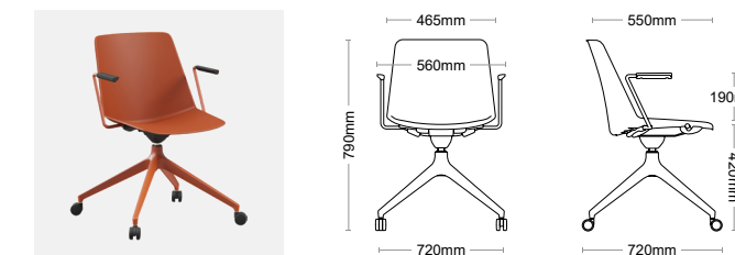
H Piramidal Rodada c/ Apoio de Braço - Pyramidal with casters and armrest Piramidal con ruedas y reposabrazos - Pyramidal avec roulettes et accoudoir
