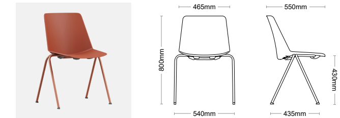
D Trenó c/ Apoio de Braço - Sled with Armrest Trineo con reposabrazos - Luge avec accoudoir
