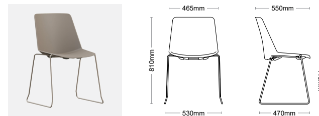
E Piramidal - Pyramidal Piramidal - Pyramidal
