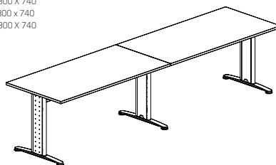
SECRETÁRIA DUPLA 2800 X 800 X 740 | 3600 X 800 X 740 3200 X 800 X 740
