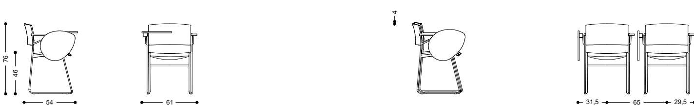
Zinia con tavoletta - Zinia chair with tablet
